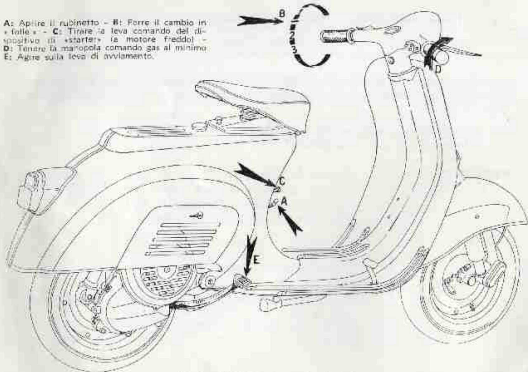
Fig. 6 - Operazioni per avviare la moto
