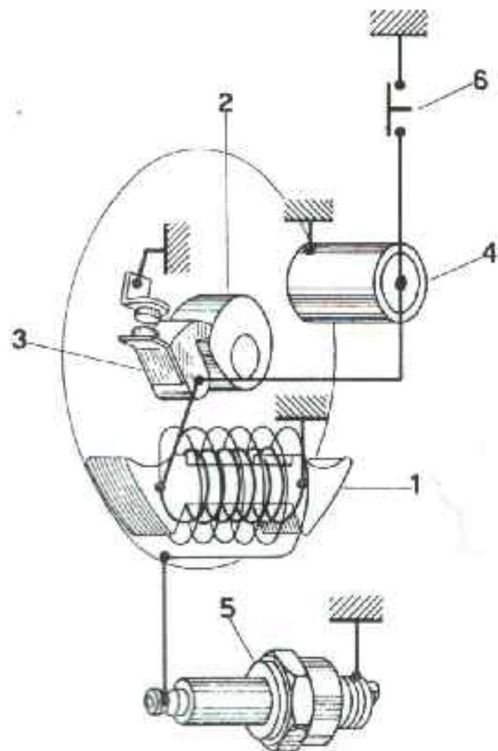
Fig. 15 - Schema dell'accensione
