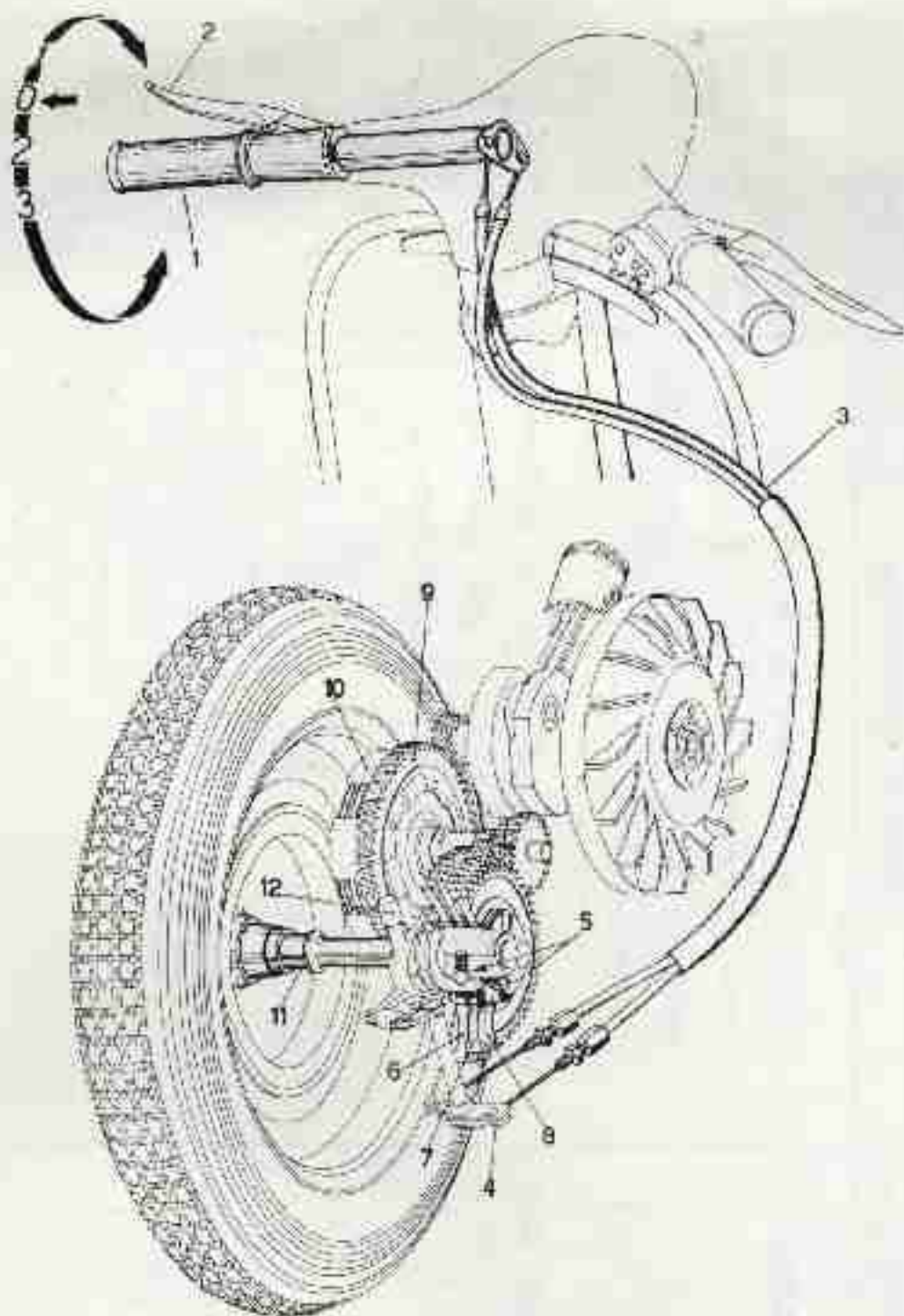
Fig. 7 - Schema del cambio
