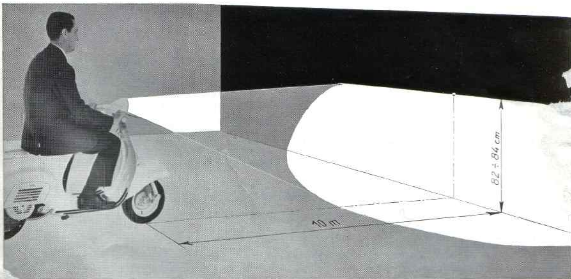
Fig. 14 - Schema orientamento proiettore
