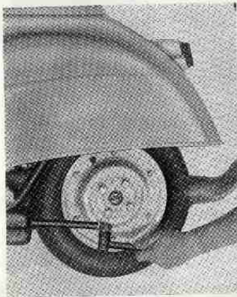
Fig. 9 - Svintaggio ruota dal «collo»
