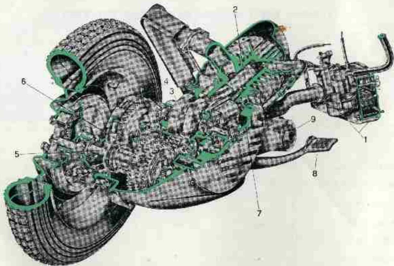
Fig. 3 - Sezione del motore
